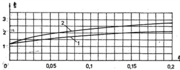
Фиг. 4. Коефициент на динамичност \xi
