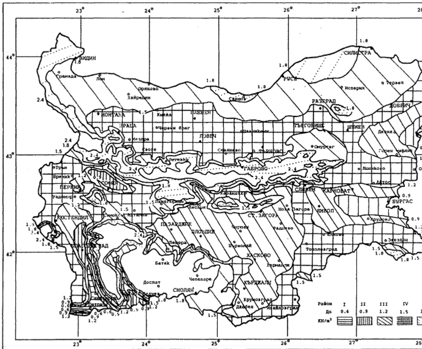
Карта за райониране на територията на страната по нормативни стойности на натоварването от сняг върху терена s_t (кН/м 2 )
