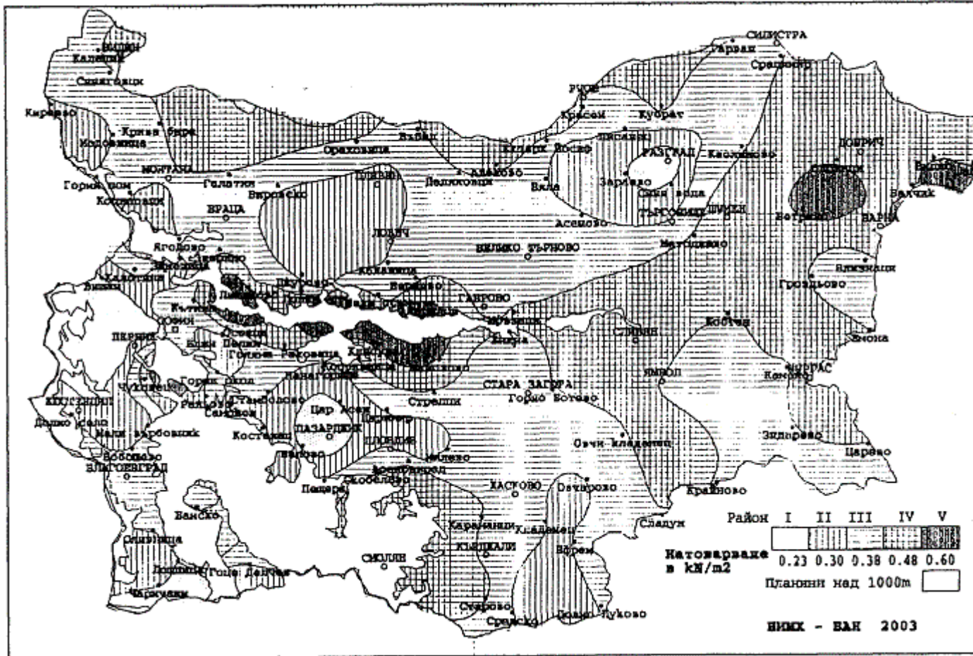
Карта за райониране на територията на страната по нормативни стойности на налягането от вятър w_m ( kN/m^2 )
