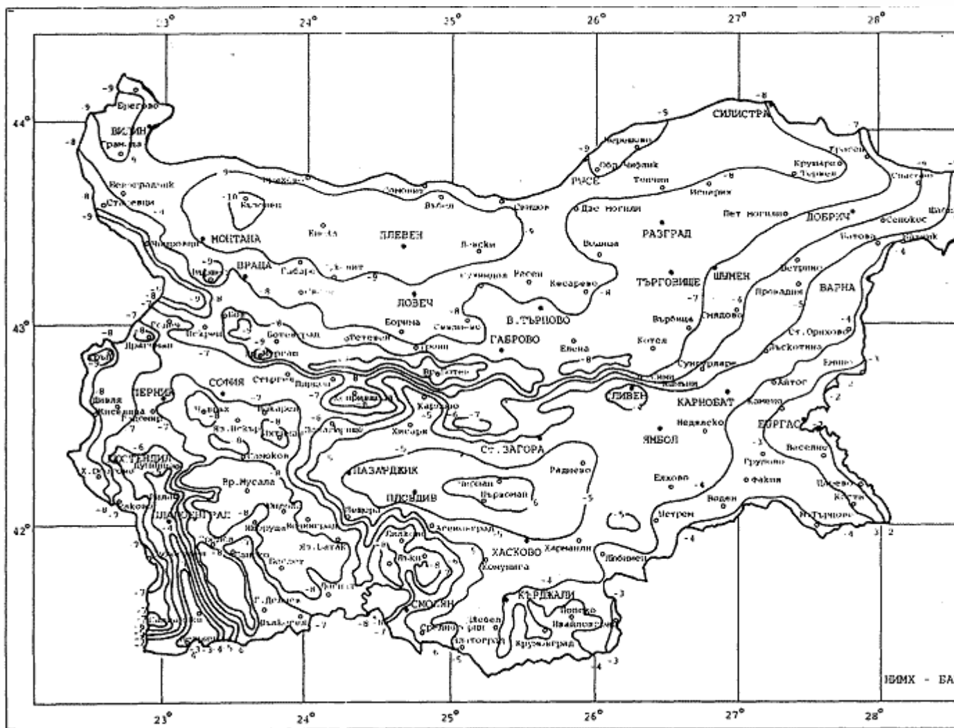
Карта № 4. Средноденонощна температура на външния въздух за януари ( t_1 )
